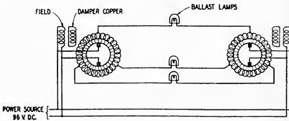
FIG. 1. Multiduty motor system.
